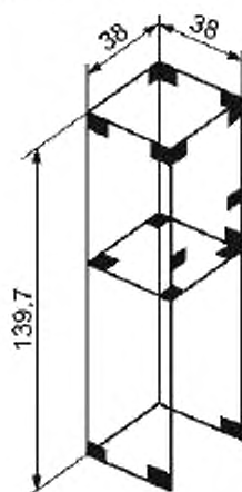
а) Корзинка из проволоочной сетки
