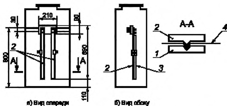
Рисунок 5 — Испытательная камера
