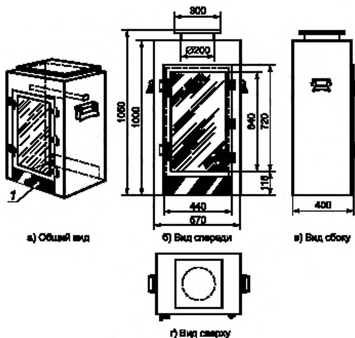
Рисунок 5 — Испытательная камера
