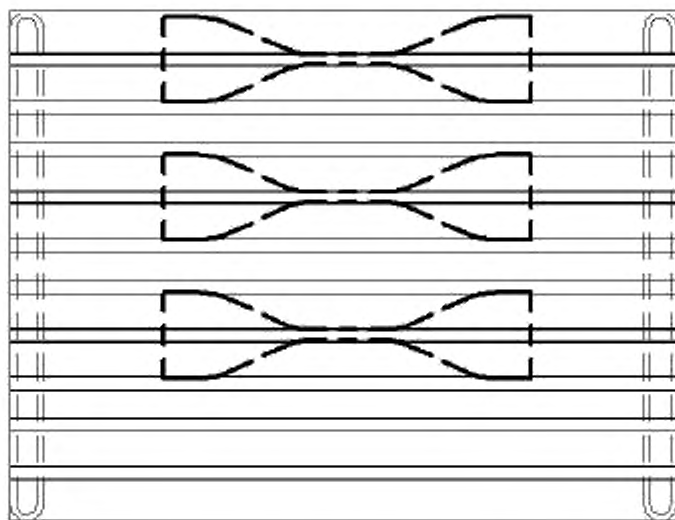
Рисунок 1 — Вырубка образцов из пазов прокладки
