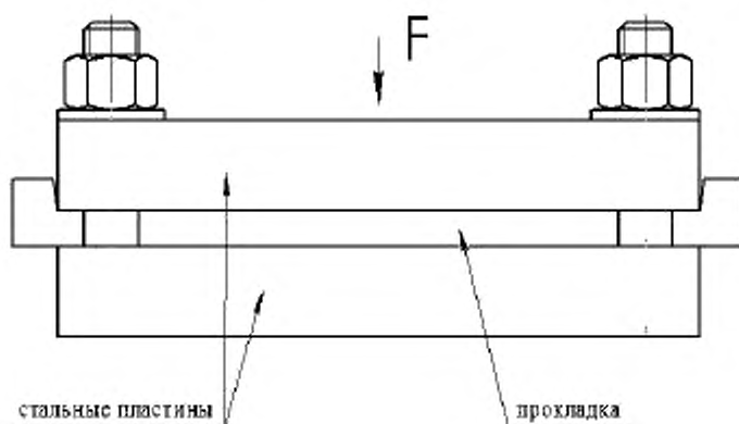
Рисунок 6 — Струбцина для проведения испытаний
