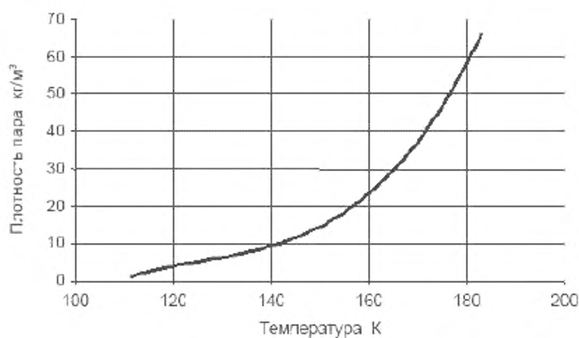
Рисунок А.3 – Плотность насыщенного пара метана
