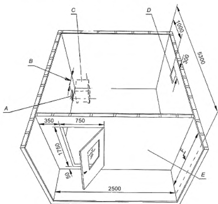
А — вход воздуха; В — регулируемое расстояние; С — нагреватель для сауны ; D — выход воздуха; Е — передвижная стена; F — 1900, 2100 или 2300 мм
