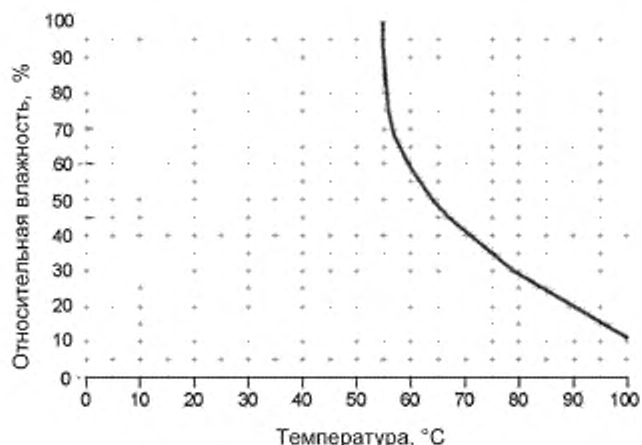
Рисунок 102 — Характеристика температуры/относительной влажности при ненормальной работе
