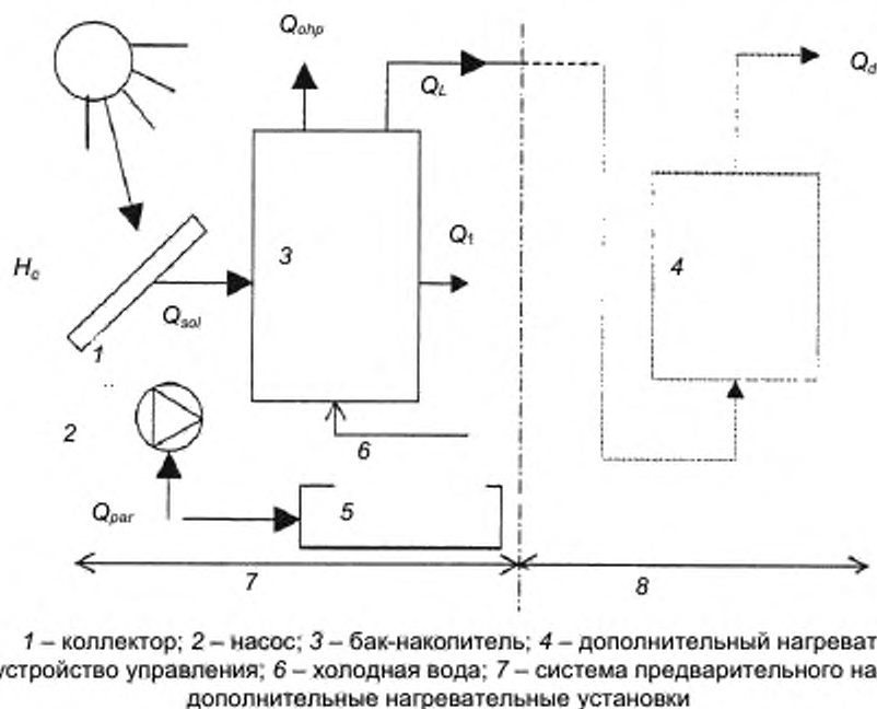
Рисунок 3 – Энергетический баланс для солнечных систем предварительного нагрева
