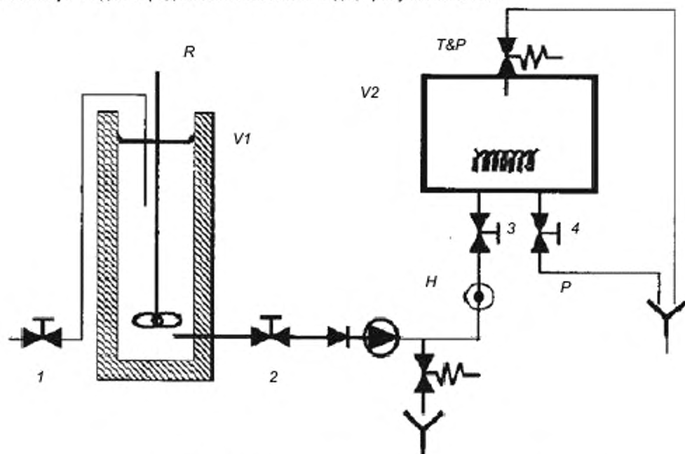
Рисунок Г.1 – Комплект для испытания клапана термостата
