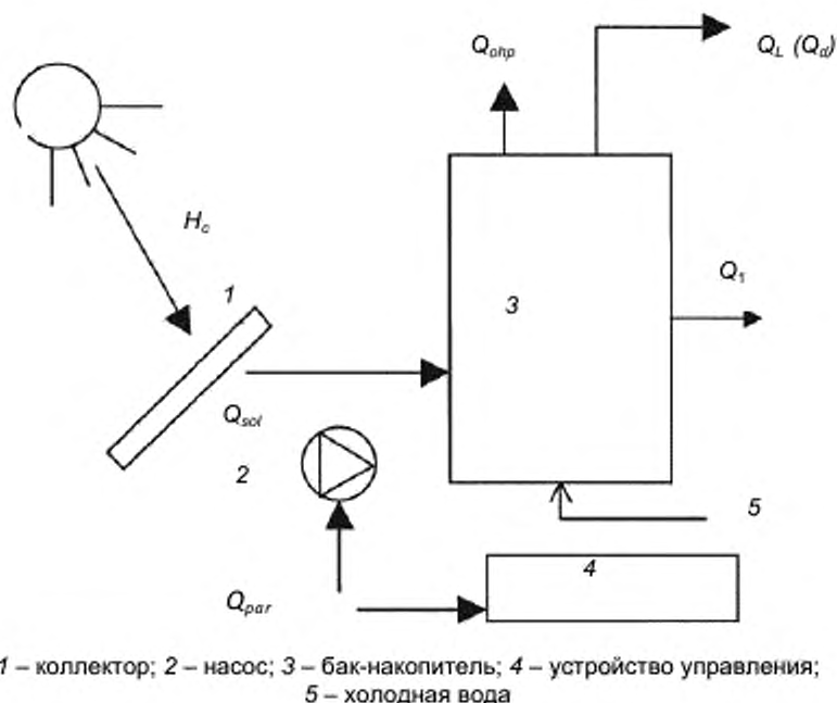
Рисунок 2 – Энергетический баланс для солнечной системы теплоснабжения
