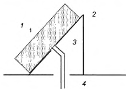
1 – солнечная система БГВ; 2 – пристройка к крыше; 3 – температура внутри помещения; 4 – трубы системы, через отверстие в крыше Рисунок В.4 – Солнечная система БГВ, смонтированная на наклонной крыше с тепловым контактом с воздухом внутри помещения
