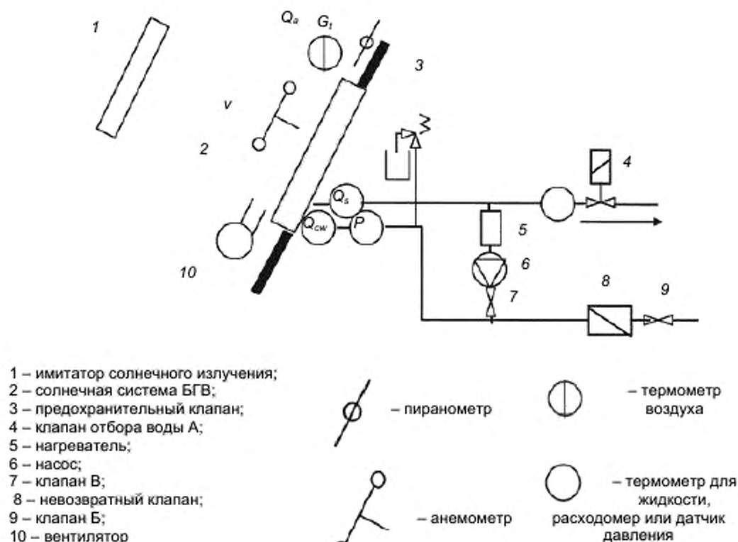
Рисунок В.6 – Схема структуры испытания
