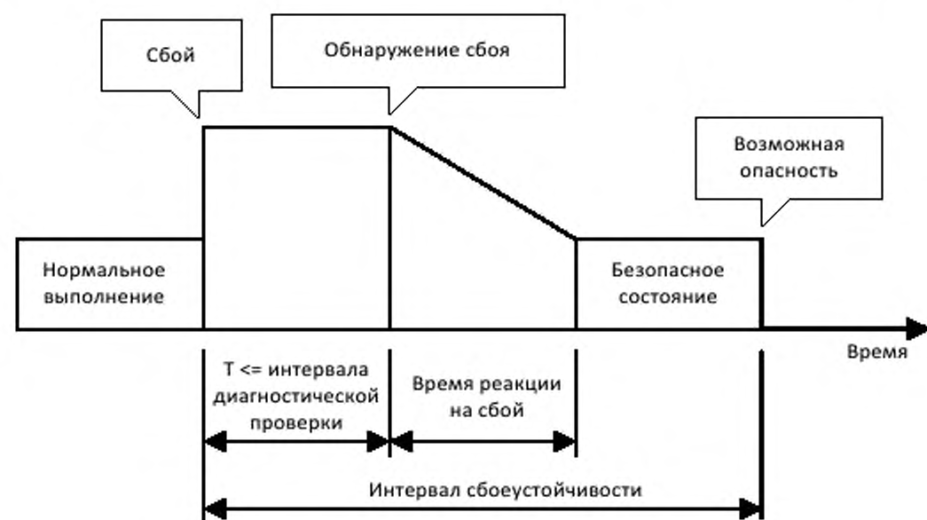
Рисунок 4 — Время реакции на сбой и интервал сбоеустойчивости
