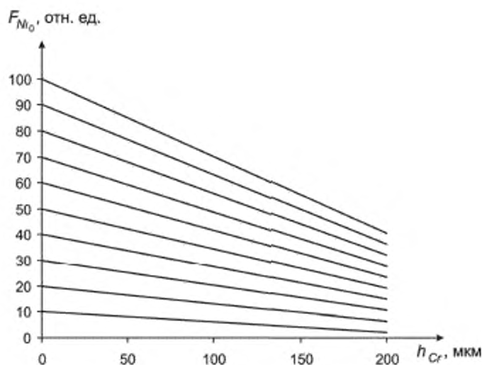
Рисунок 3 — Номограмма для определения толщины хромового покрытия
