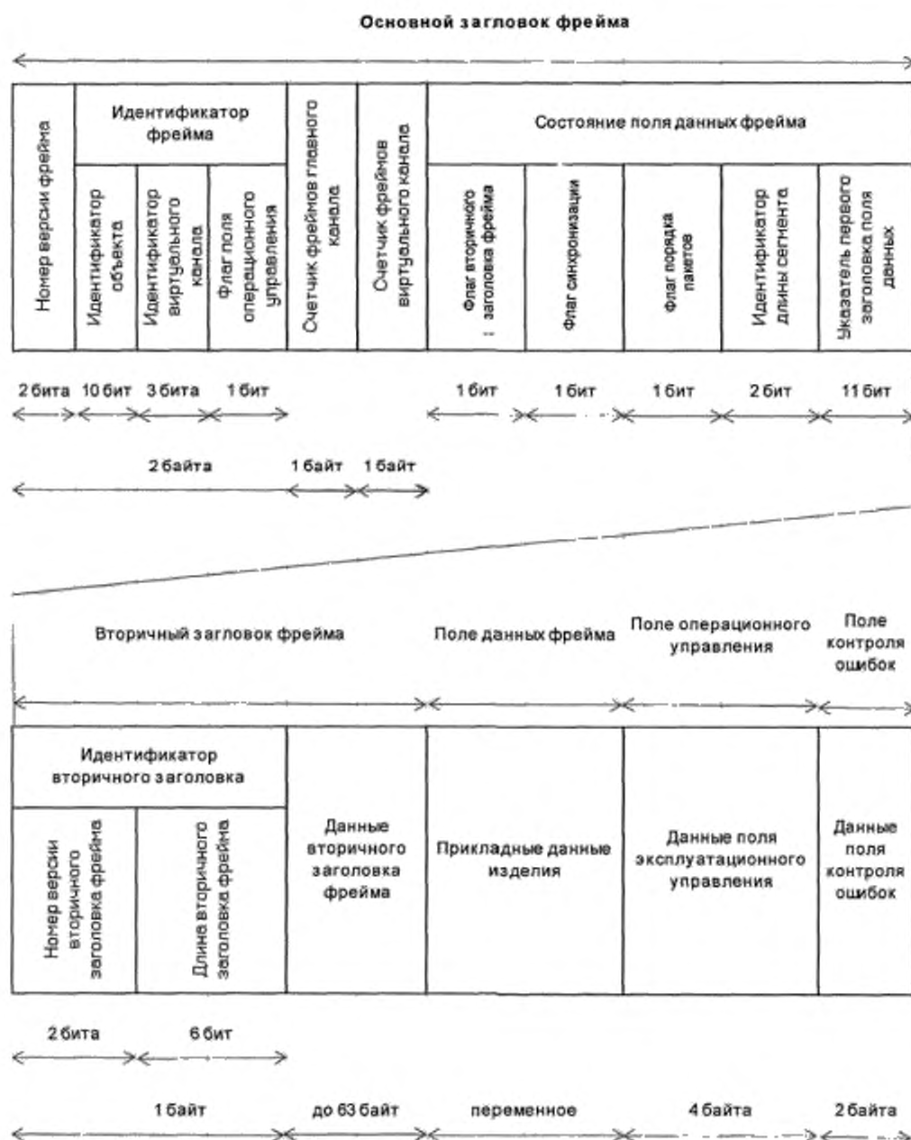
Рисунок 9 — Структура фрейма передачи
