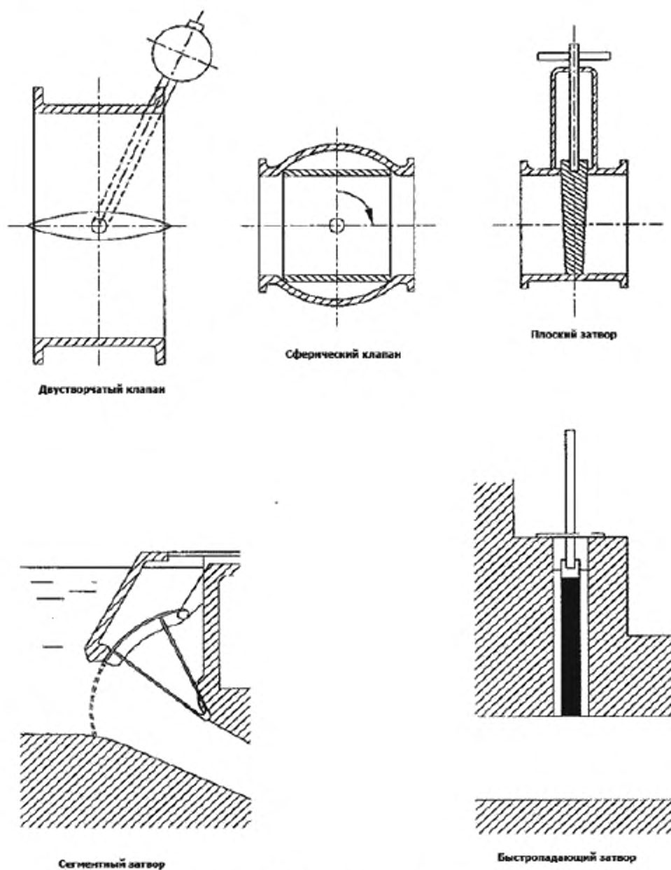
Рисунок ДА.7 –Примеры затворов
