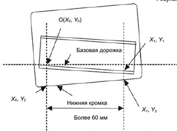
Рисунок 3 – Методика измерения наклона
