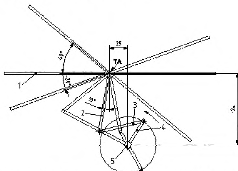
Рисунок 10 — Асимметричный (60:40) кривошипно-шатунный механизм по 3.4.2. Диапазон наклона от минус 20^\circ (контакт пятки) до плюс 40^\circ (отрыв носка)
