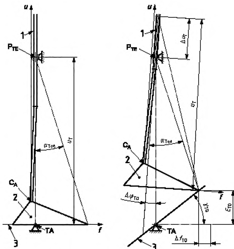
Рисунок 22 – Иллюстрация влияния А–Р смещения \Delta f на угловое перемещение \Delta\varphi испытываемого образца относительно «внешней» верхней точки приложения нагрузки P_{TE} в сборке согласно 3.3.3
