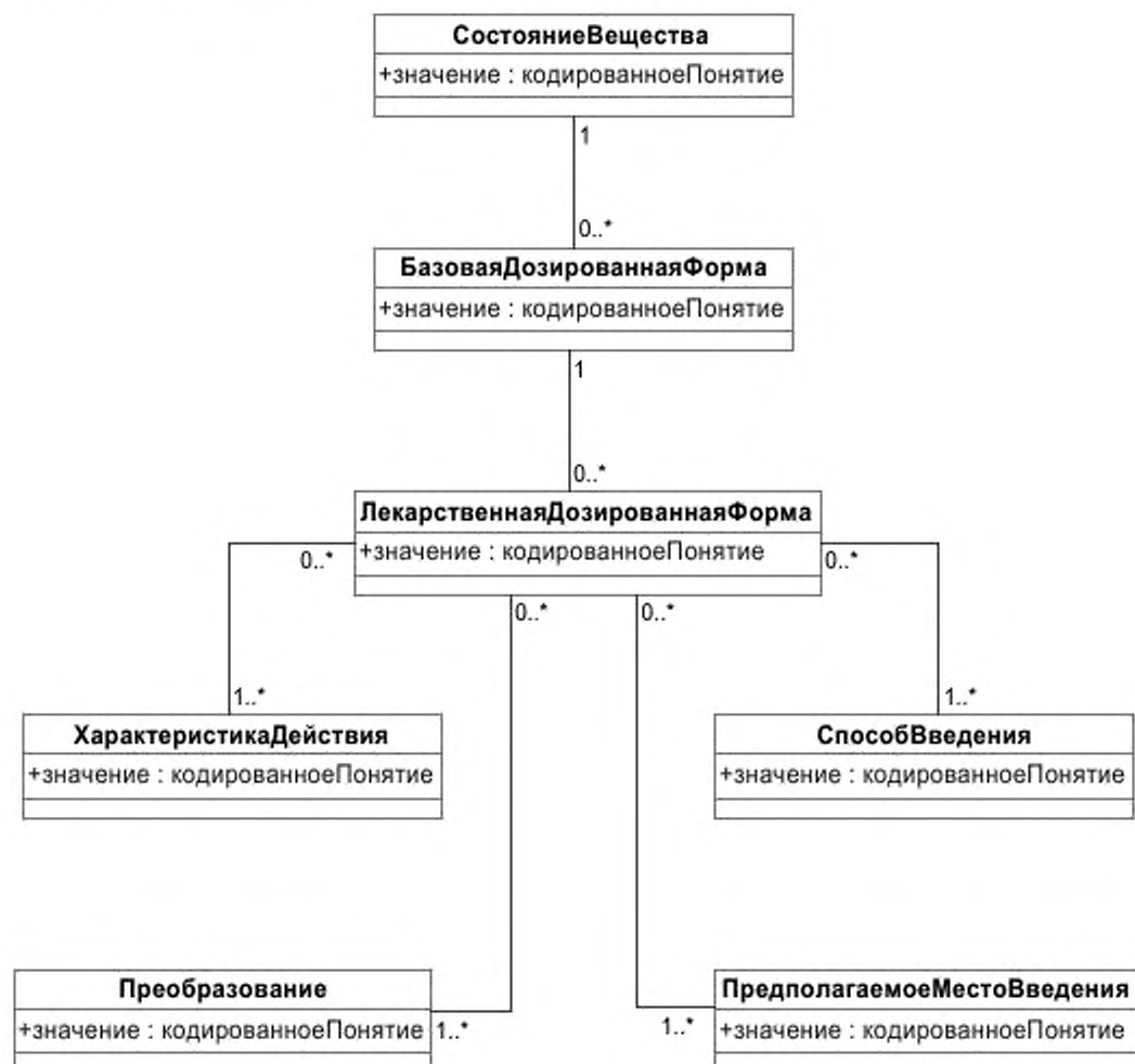
Рисунок 5 – Концептуальная диаграмма класса «ЛекарственнаяДозированнаяФорма»
