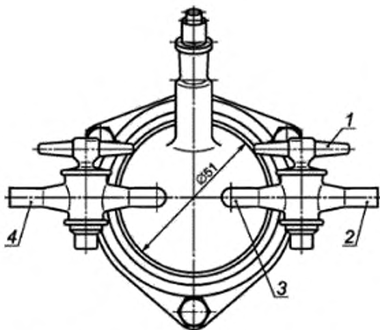
1 — запорный клапан; 2 — выпускное отверстие; 3 — трубка для отбора жидкости или газа; 4 — выпускное отверстие
