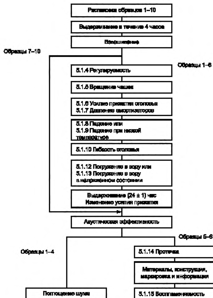
Рисунок В.1 — Блок-схема испытаний наушников с оголовьем
