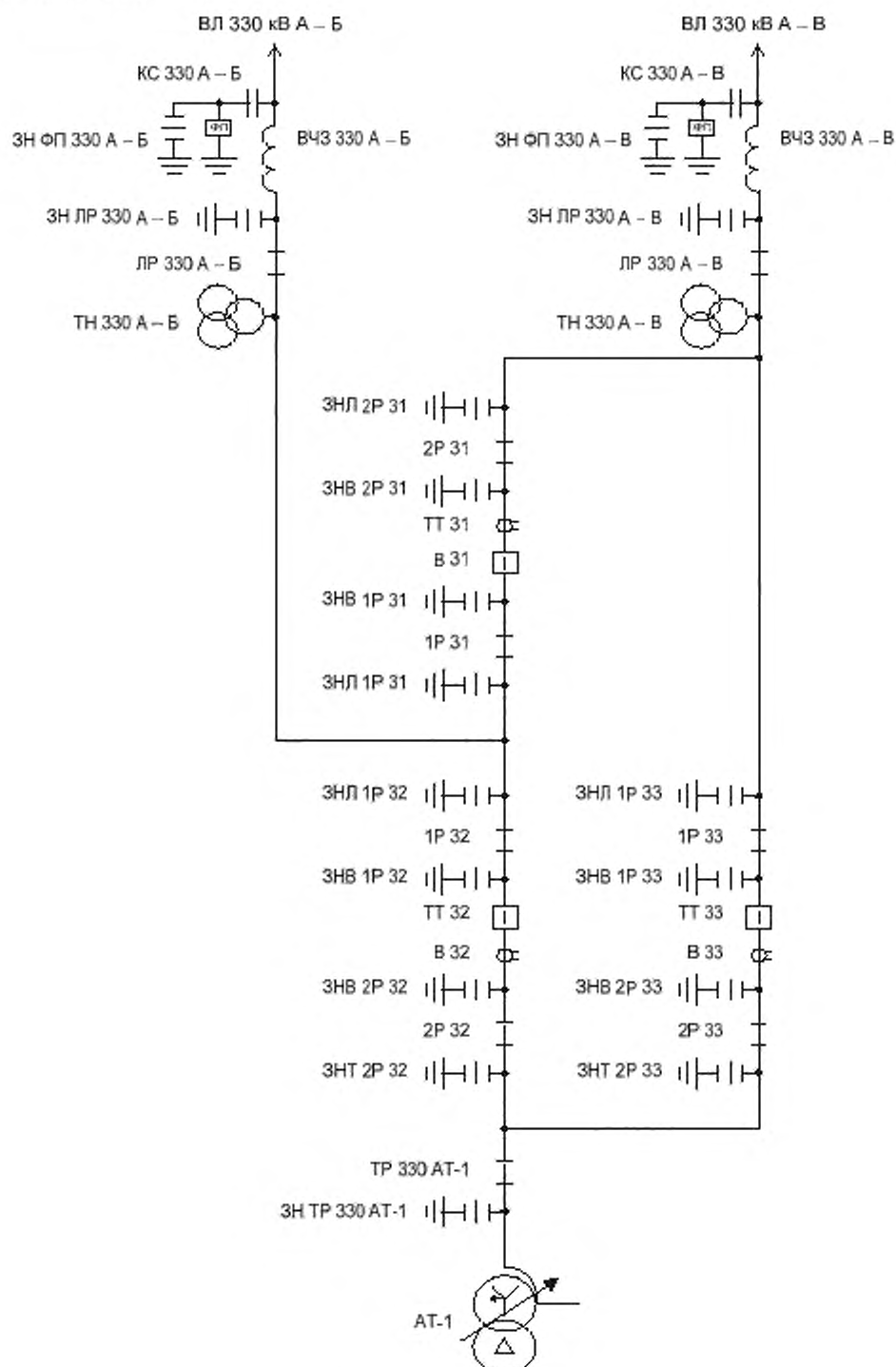
Рисунок Б.3 – Схема РУ 330 кВ типа «треугольник»
