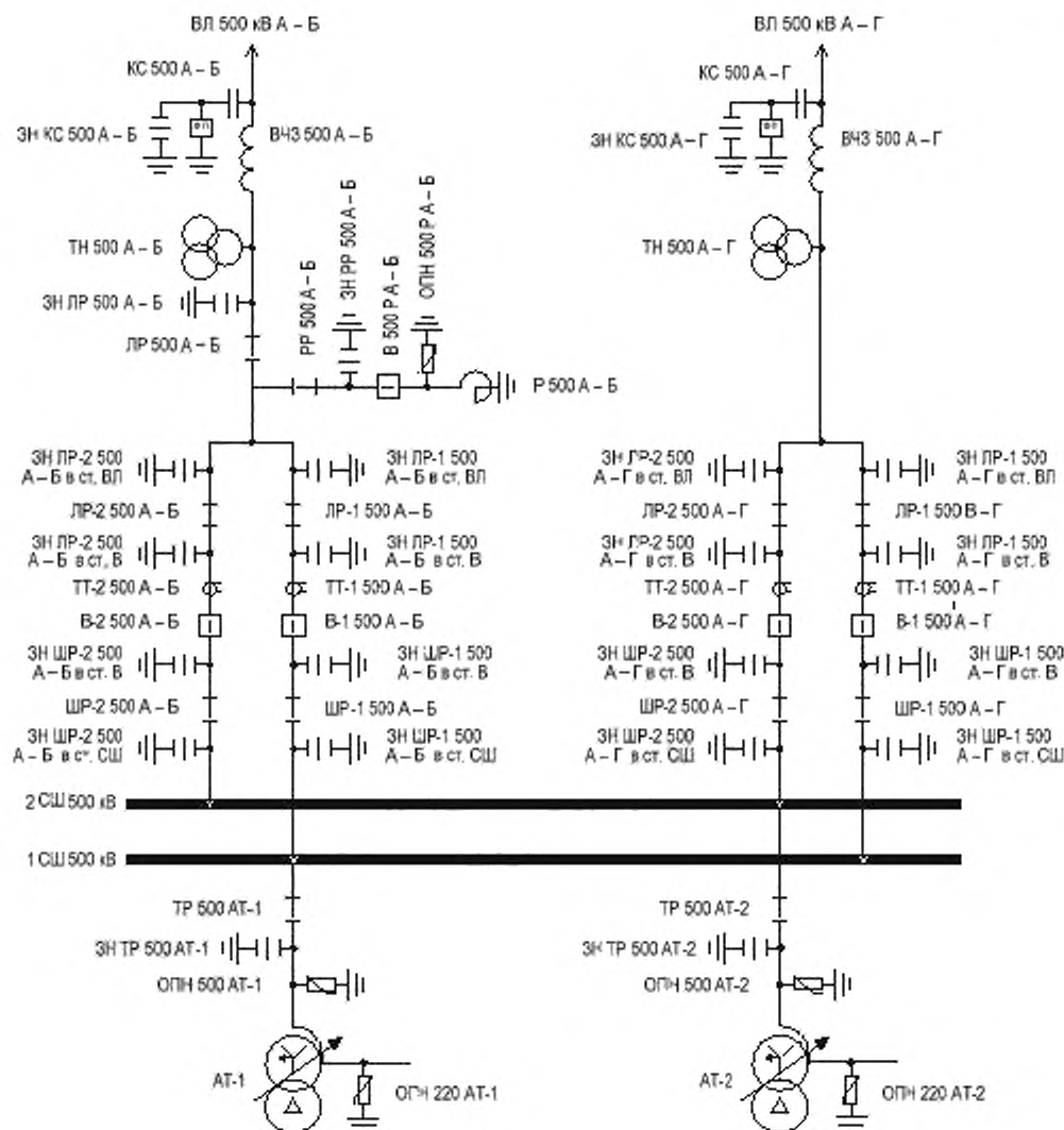
Рисунок Б.2 – Схема РУ 500 кВ типа «трансформаторы – шины» с присоединением линий через два выключателя
