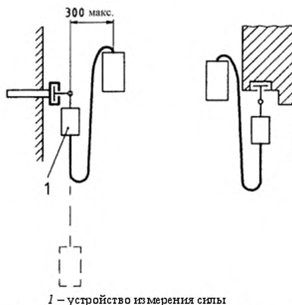
1 – устройство измерения силы Рисунок 11 – Проверка динамической прочности на анкерных устройствах с жесткой горизонтальной направляющей
