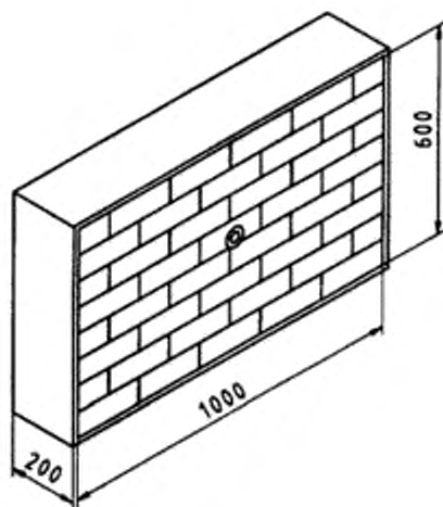
Рисунок 3 – Минимальный размер кирпичной кладки
