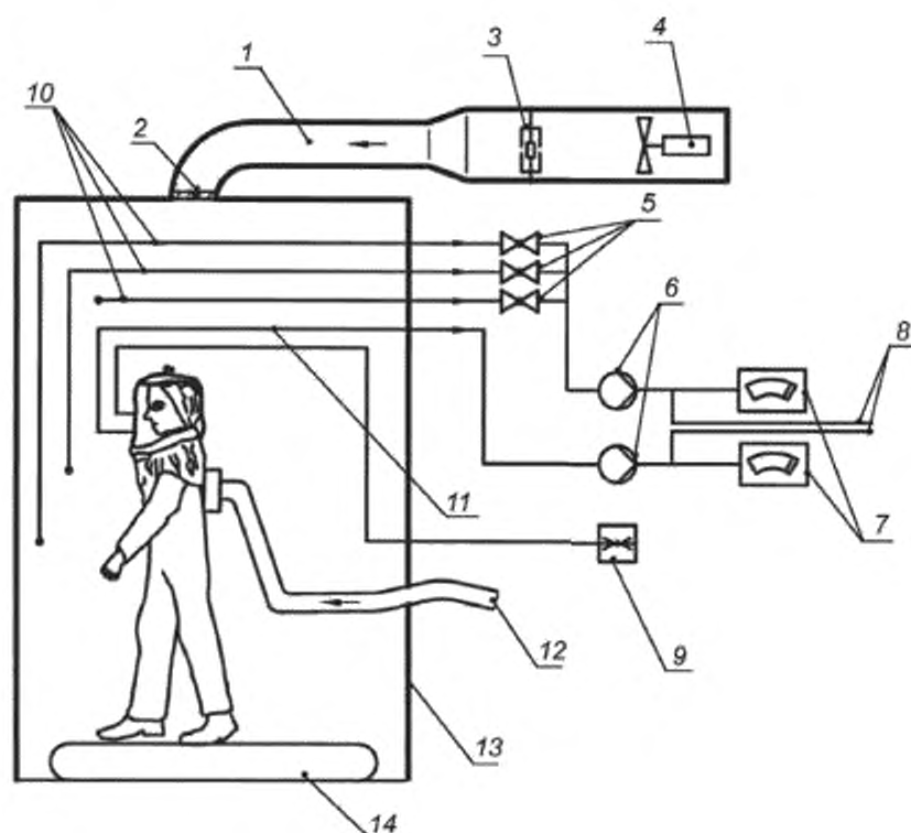
1 — воздуховод; 2 — заслонка; 3 — подача аэрозоля гексафторида серы; 4 — вентилятор; 5 — клапаны; 6 — насосы; 7 — детекторы гексафторида серы; 8 — дополнительный подвод воздуха; 9 — манометр; 10 — пробы воздуха из испытательной камеры; 11 — пробы воздуха из зоны дыхания; 12 — подача пригодного для дыхания воздуха; 13 — испытательная камера; 14 — беговая дорожка
