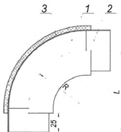
1 – стальной отвод; 2 – стальной патрубок; 3 – ППМ изоляция; R – радиус отвода; L – длина плеча отвода
