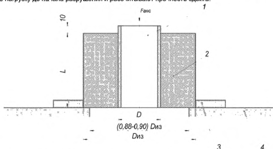
1 – стальная труба; 2 – ППМ изоляция; 3 – направляющая; 4 – упор; L – длина образца; D – диаметр стальной трубы; Диз – диаметр изоляции; F_{акс} – осевая нагрузка
