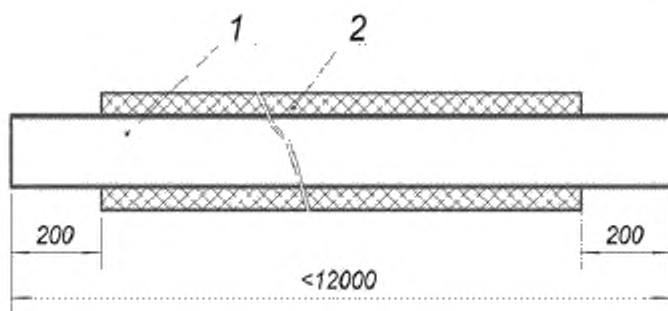
1 – стальная труба; 2 – ППМ изоляция
