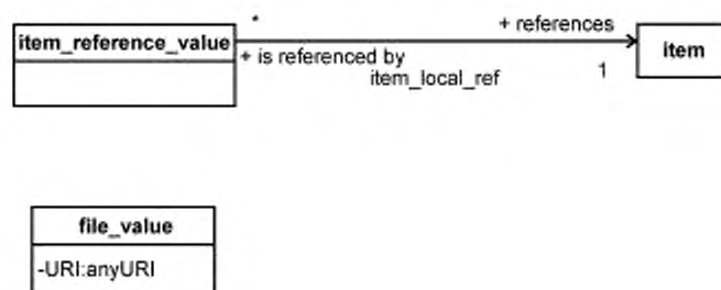
Рисунок 13 — Диаграмма класса UML для подмодели ссылочного значения
