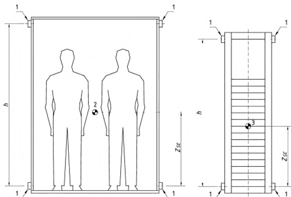
1 - башмак или контрольный башмак; 2 - центр тяжести кабины (рассчитанный с учетом массы Q_{SE} ); 3 - центр тяжести противовеса или уравновешивающего груза;
