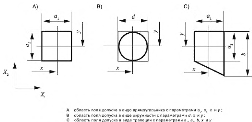
Рисунок 1 – Примеры областей поля допуска в двумерном пространстве для двумерной величины (x_1, x_2)^T
