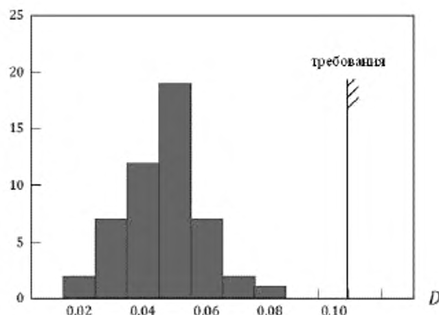
Рисунок С.4 — Гистограмма значений характеристики D
