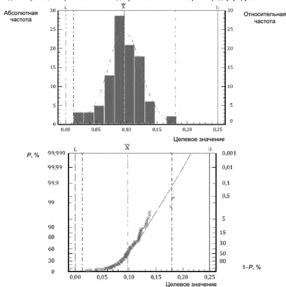
Рисунок 9 – Гистограмма и график вероятности
