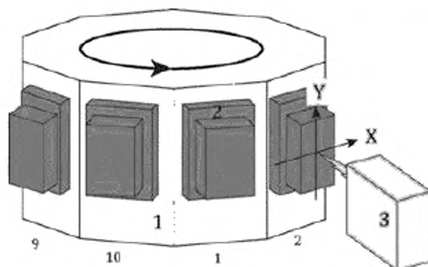
1 поворотный стол; 2 зажимное приспособление; 3 обрабатывающий центр
