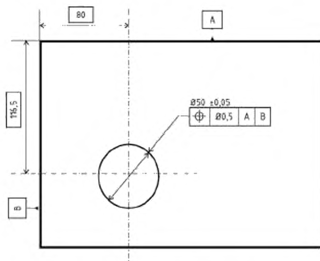
Рисунок 6 — Схема положения отверстия на детали
