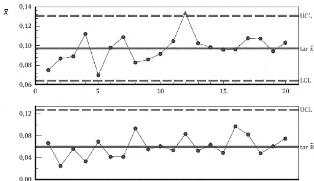
Рисунок 10 – Контрольная карта
