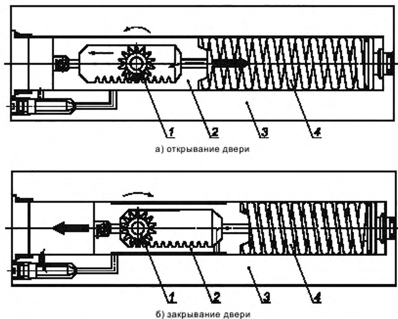
Рисунок В.1 — Пример конструкции доводчика
