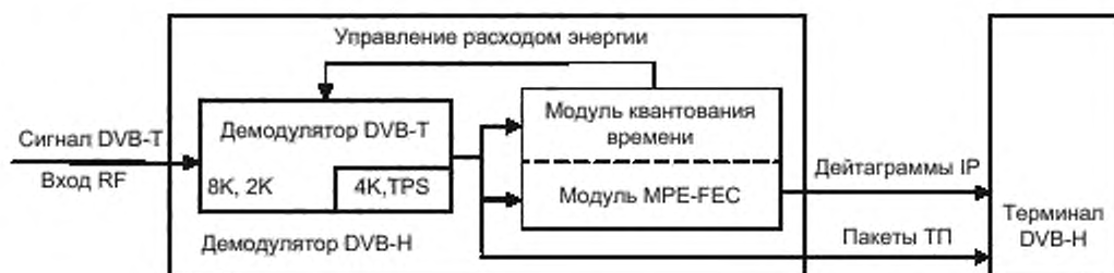
Рисунок 1 — Концептуальная структура приемника DVB-H
