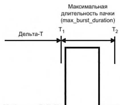
Рисунок 7 — Максимальная длительность пачки
