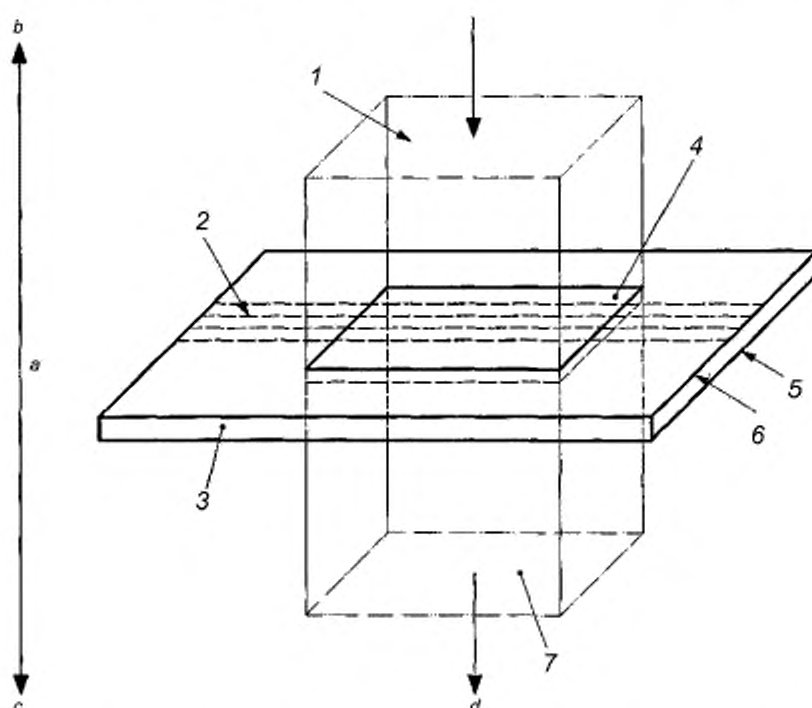
1 — поток воздуха; 2 — перфорированная зона; 3 — испытуемая проба; 4 — измеряемая поверхность пробы площадью 2 см 2 ; 5 — внутренняя поверхность; 6 — наружная поверхность; 7 — поток воздуха; а — перепад давления; b — высокое давление; c — низкое давление; d — направление воздушного потока
