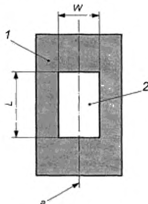
1 — испытываемая проба; 2 — зона измерения испытываемой пробы в держателе; L — длина измеряемой поверхности; W — ширина измеряемой поверхности; а — осевая линия испытываемой пробы
