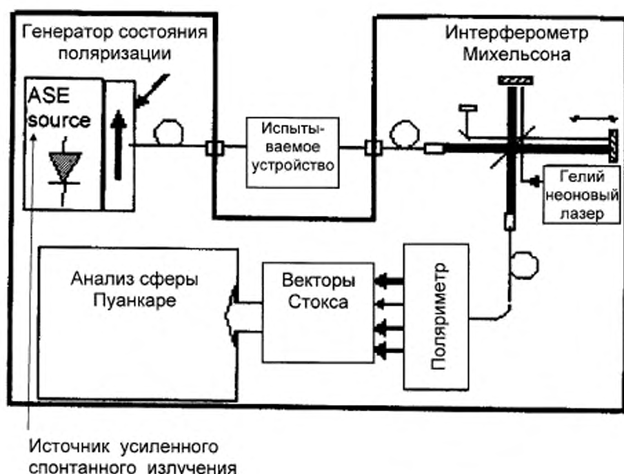
В.1b – широкополосный источник (JME)
