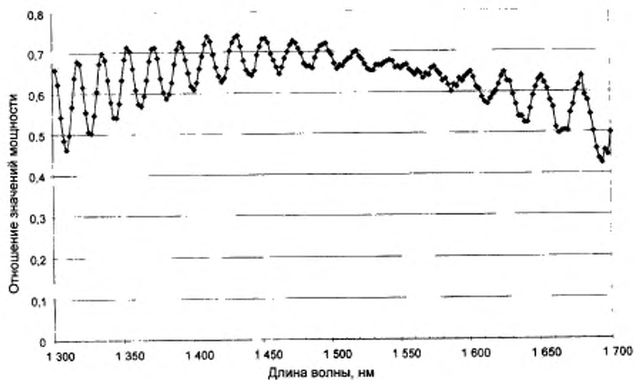
А.2а – незначительная связь мод
