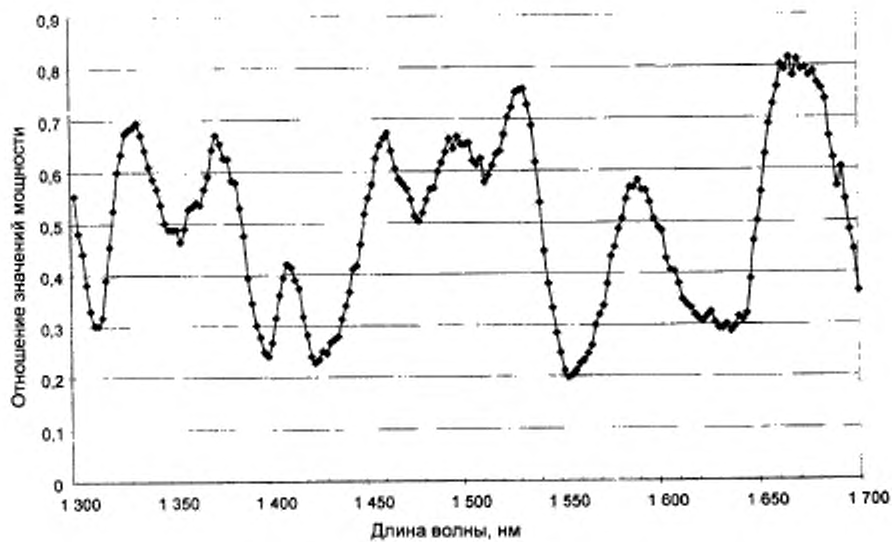
А.2б – случайная связь мод
