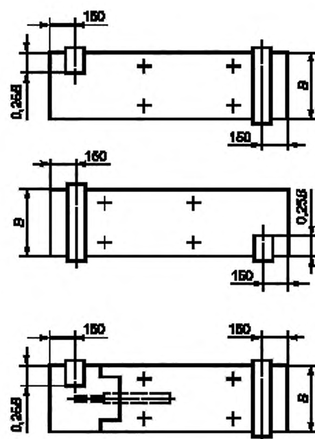
Рисунок А.5 — Схемы нагружения жесткой балки перекрытия и перекрытия с гидropоджимной консолью при испытании на изгиб с кручением
