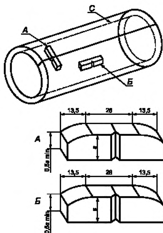
А — поперечный образец в зоне сварного шва; Б — продольный образец по телу трубы или муфты; С — сварной шов электросварных труб; x — толщина стенки трубы
