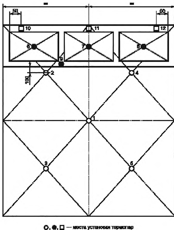
Рисунок А.4 — Схема установки термопар на необогреваемой поверхности перегородки
