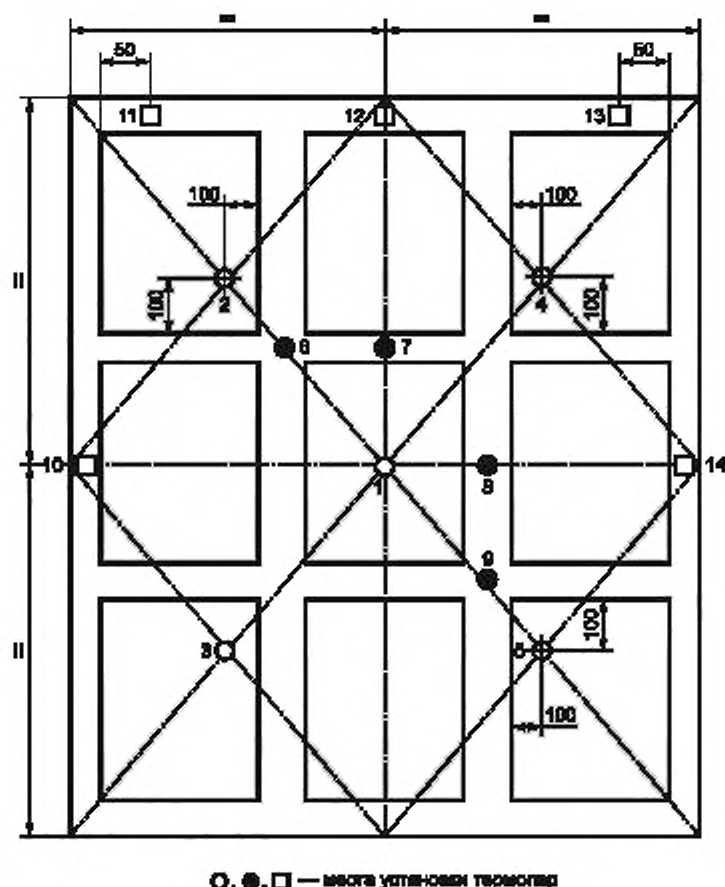
Рисунок А.2 — Схема установки термопар на необогреваемой поверхности перегородки
