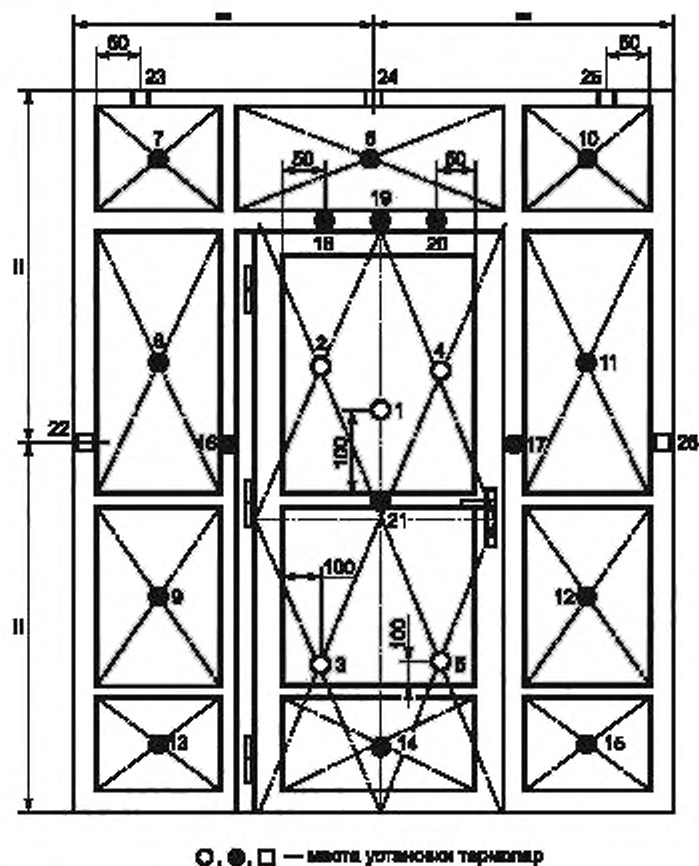
Рисунок А.10 — Схема установки термодпар на необогреваемых поверхностях перегородки и вмонтированного в нее однопольного дверного блока со светопропускающими и глухими элементами
