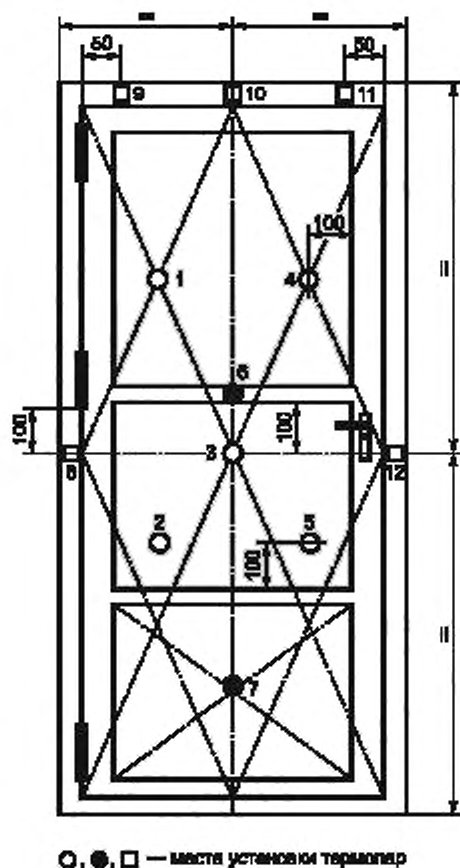
Рисунок А.5 — Схема установки термопар на необогреваемой поверхности однопольного дверного блока
