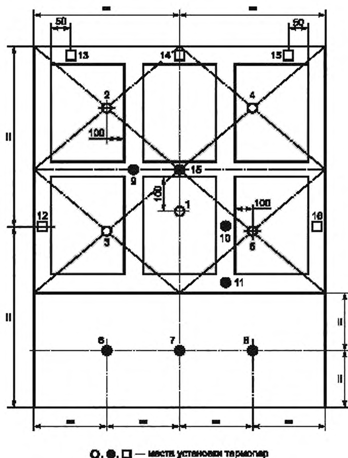
Рисунок А.3 — Схема установки термопар на необогреваемой поверхности перегородки
