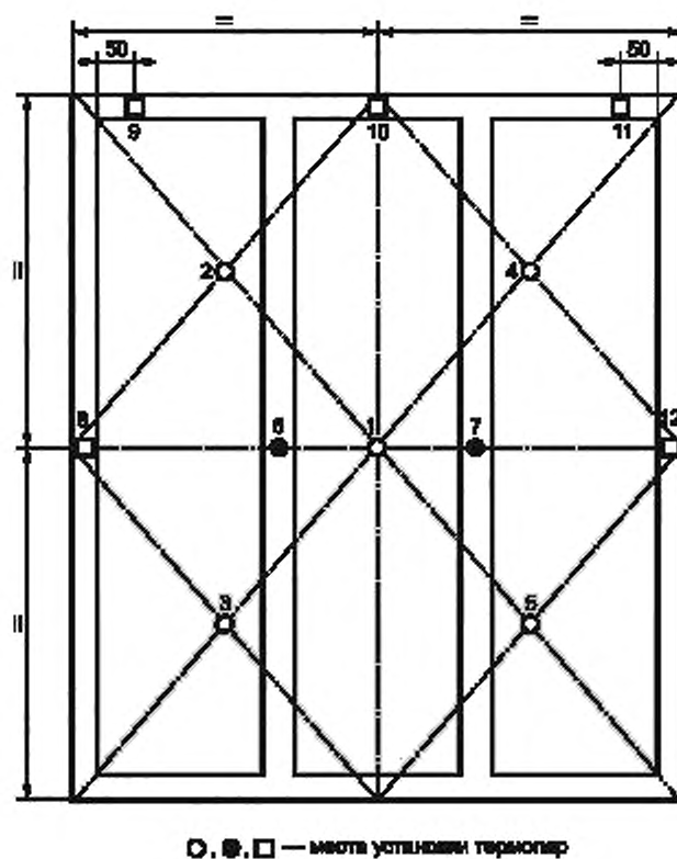
Рисунок А.1 — Схема установки термопар на необогреваемой поверхности перегородки или перекрытия
