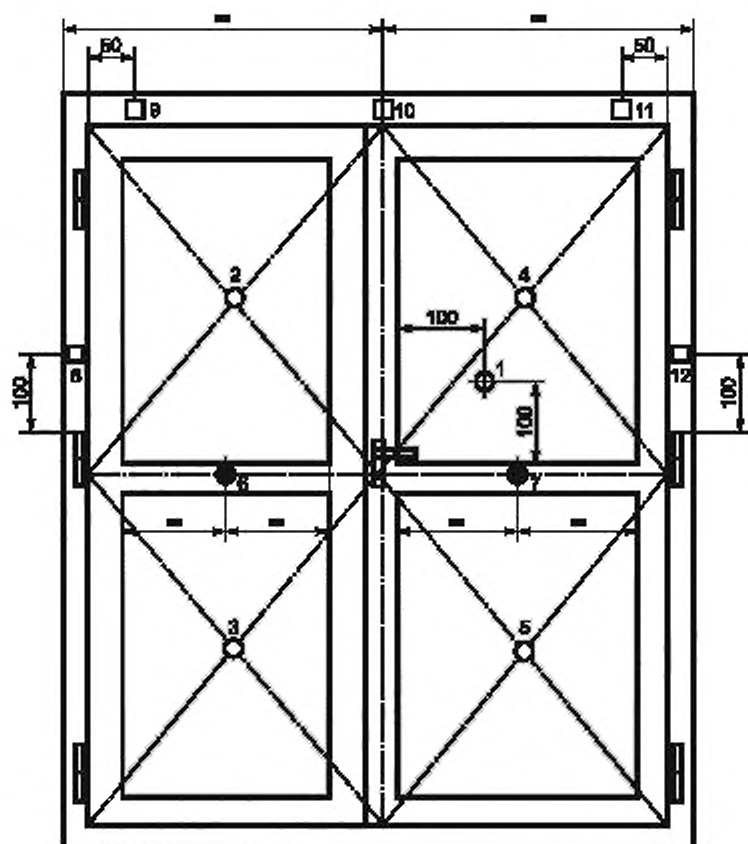
Рисунок А.7 — Схема установки терморазрыв на необогреваемой поверхности двухлопного дверного блока
