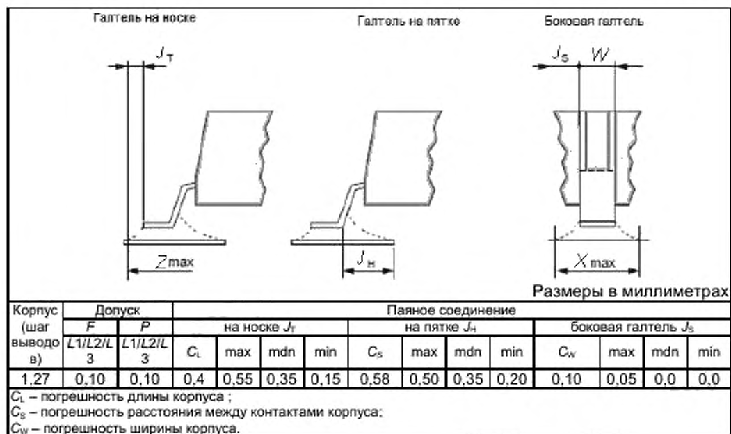
Рисунок 11 – Выступ паяного соединения (см. IEC 61188-5-1, таблицы 2 и 3)
