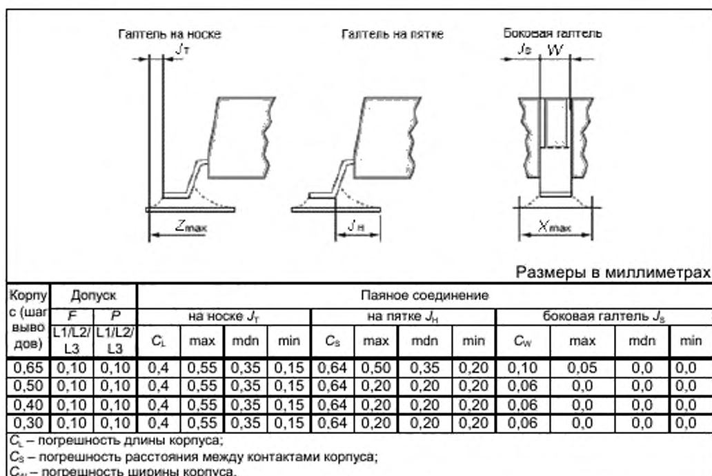
Рисунок 3 – Выступ паяного соединения (см. IEC 61188-5-1, таблицы 2 и 3)
