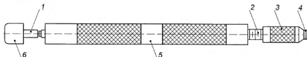
1 – индикаторный стержень; 2 – плунжер; 3 – зажим; 4 – наконечник; 5 – корпус; 6 – колпачок
