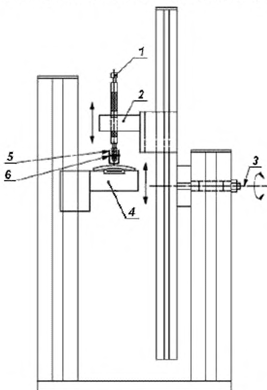
1 – истирающий инструмент; 2 – держатель инструмента; 3 – ось вращения; 4 – держатель испытываемой линзы, 5 – марля; 6 – устройство крепления марли
