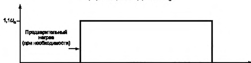
Профиль испытательного напряжения U_T главной цепи
