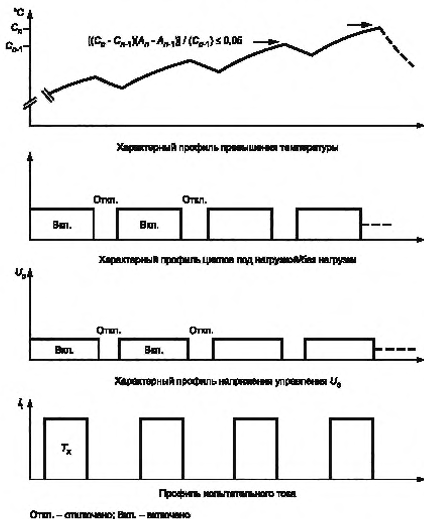
Рисунок F.1 — Профиль испытания на тепловую стабильность
