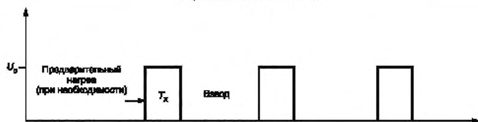
Профиль напряжения управления U_0
