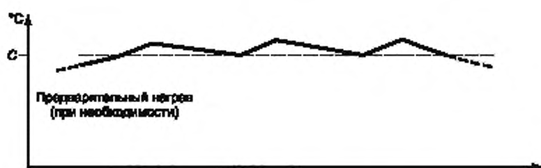
Характерный профиль повышения температуры
