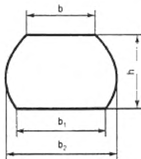
Рисунок 2 — Поперечное сечение бруса вида Б
