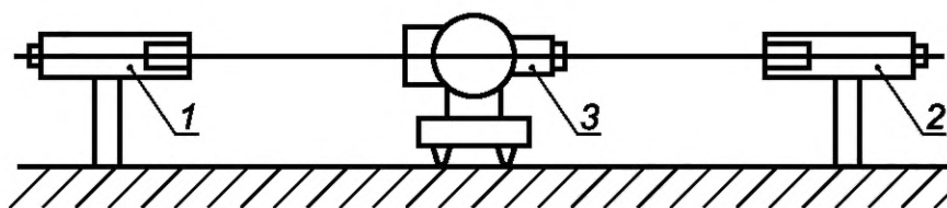
1, 2 — коллиматоры; 3 — теодолит
