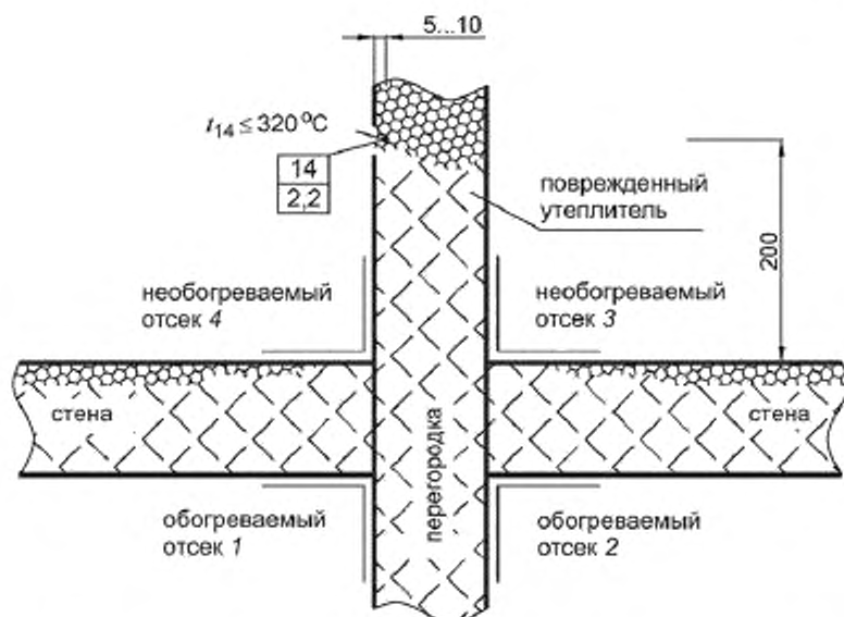
Рисунок Д.6 — Температура в контрольной точке 14 и схема распространения огня из отсеков 1 и 2 по строительным конструкциям между отсеками 1—4, вид сверху
