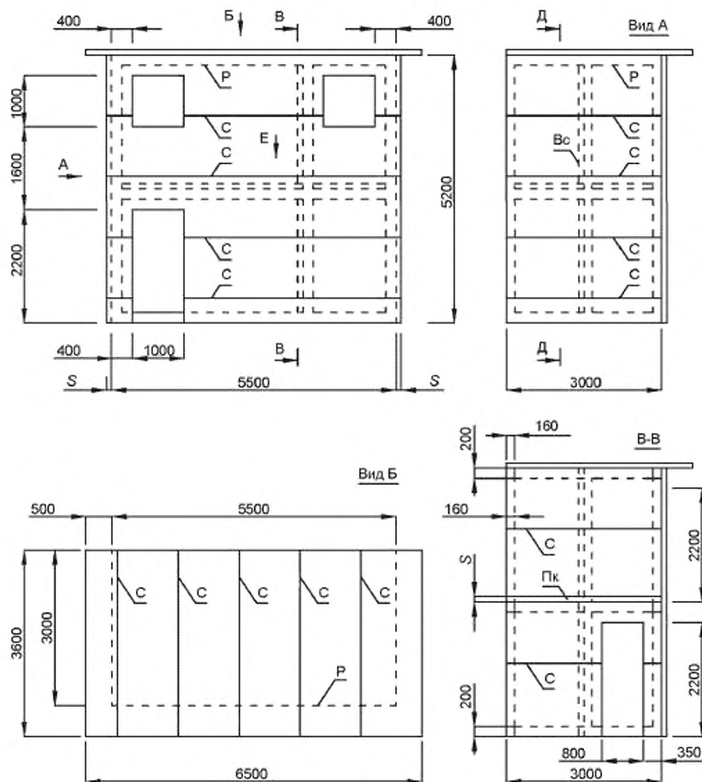
Рисунок Г.1 — Фрагмент здания: фасад, вид сбоку (А); вид сверху (Б); разрез перед перегородкой (В-В); С — стыки панелей; Р — контур рамы; S — толщина панелей; Пк — перекрытие; Bs — внутренняя стена
