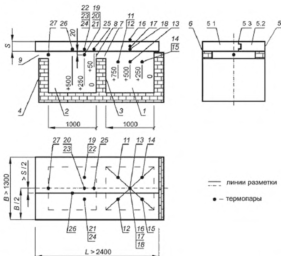
Рисунок В.2 — Схема сборки образцов и установки термодар при испытании на пожарную опасность горизонтальных конструкций из панелей (обозначения приведены на рисунке В.1)
