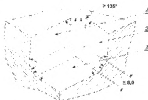
Рисунок В.4 – Соединенные поверхности в пищевой зоне
