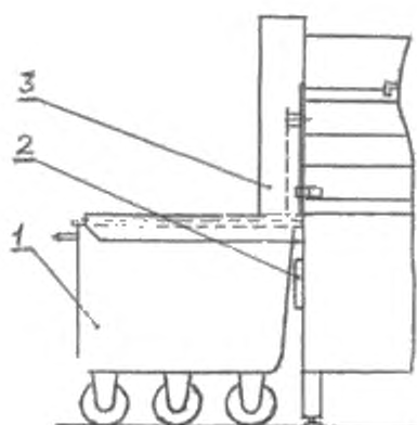
1 – тележка для нарезанного продукта, 2 – переключатель положения, 3 – разгрузочный лоток
