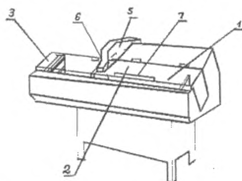
Рисунок 4 – Опасные зоны ломтерезки с разгрузочным лотком
