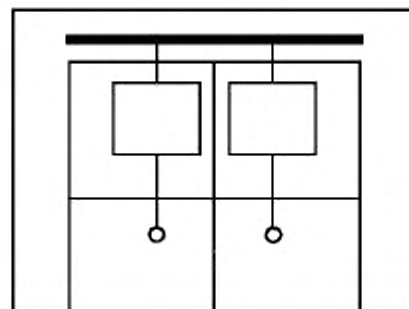
Вид 4b — Зажимы для внешних проводников в разных секциях с функциональным блоком
