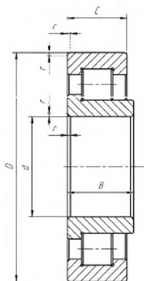
Рисунок 3 – Конструктивное исполнение 42000У с однорядковым выступающим внутренним кольцом
