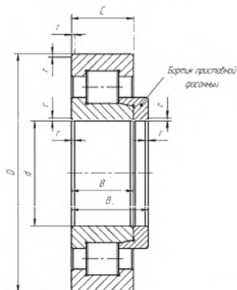
Рисунок 5 – Конструктивное исполнение 62000 с однорядковым внутренним кольцом и фасонным приставным бортиком
