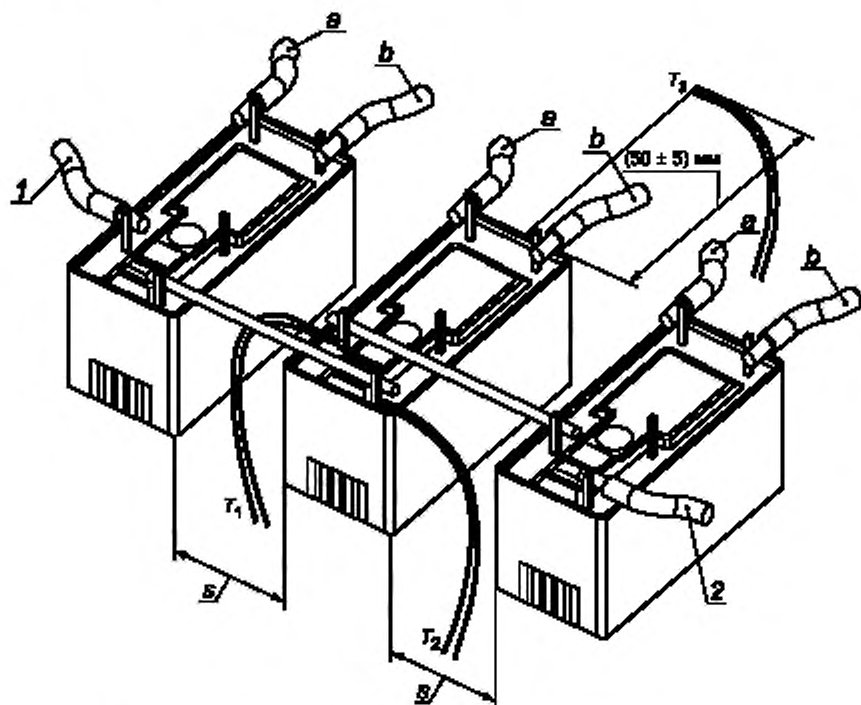
1, 2 — клеммы контактов; a, b — клеммы катушки; S — установочное расстояние; T_1 — термодатчики.
