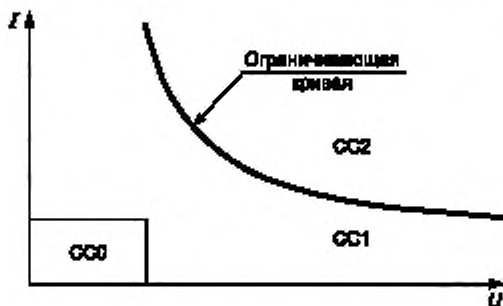
Рисунок С.3 — Категории контактных нагрузок
