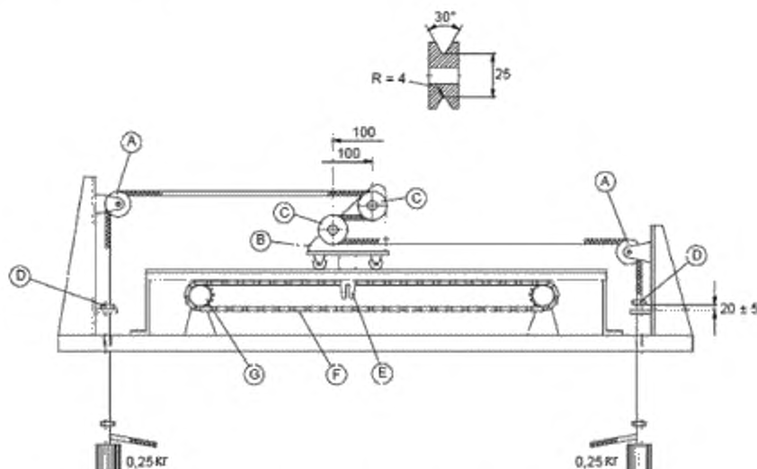
А — шкив диаметром > 50 мм; В — каретка; С — шкив с желобком; D — ограничительный зажим; E — штифт зацепления; F — цепь, имеющая шаг зацепления 12,7 мм; G — цепное колесо, имеющее 20 зубьев с диаметром делительной окружности 88,9 мм
