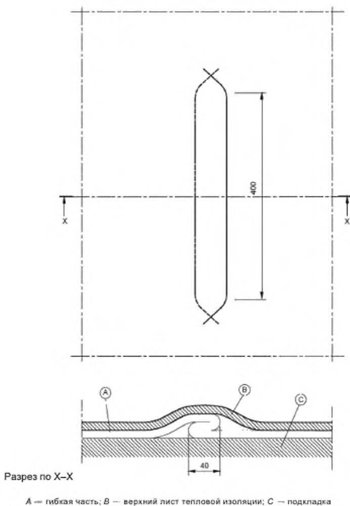
Рисунок 105 — Расположение для испытания складки тройной толщины
