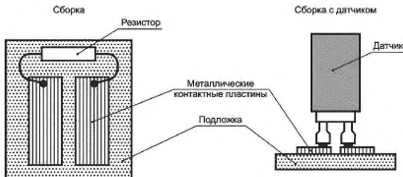
Рисунок 3 — Сборка для проверки сопротивления
