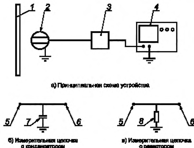
1 — заряженный объект или поверхность, 2 — сферический двухкомпонентный разрядный электрод; 3 — измерительная щуп; 4 — цифровой запоминающий осциллограф (например, с полосой пропускания 1 ГГц); 5 — контактное соединение с электродом; 6 — контактное соединение с осциллографом; 7 — конденсатор (например, 20 нФ), 8 — резистор (например, 0,25 Ом)
