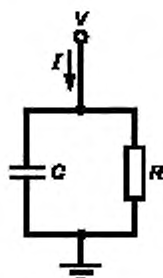
Рисунок 3 — Эквивалентная электрическая цепь заряжения проводника
