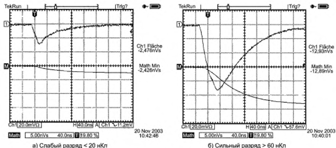
Рисунок 4 — Примеры форм импульса кистевого разряда на экране быстродействующего цифрового запоминающего осциллографа
