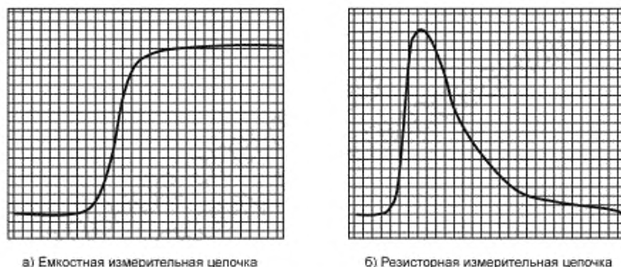
а) Емкостная измерительная цепочка
