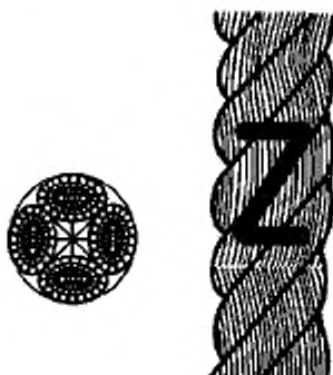
Рисунок 2- Конфигурация 4-прядного крученого каната (тип В)
