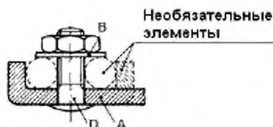
A — зафиксированная токоведущая часть; B — прижимные детали; C — прижимная деталь, защищающая от скольжения гайки по проводнику; D — болт (винт)
