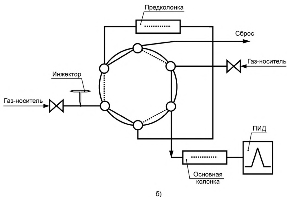
Рисунок 3 — Схема прямой (а) и обратной (б) продувки предколонки газового хроматографа
