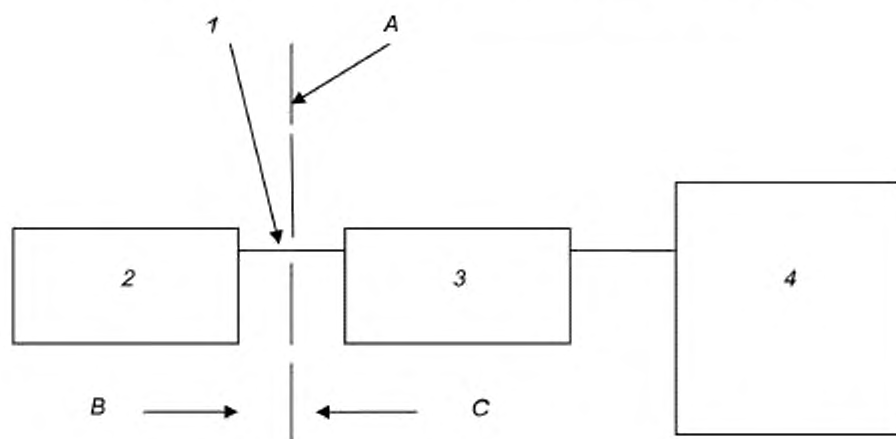
Схема соединения системы сигнализации здания с лифтом
