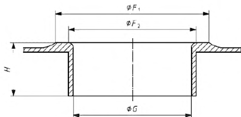
Рисунок А.2 — Заливная горловина
