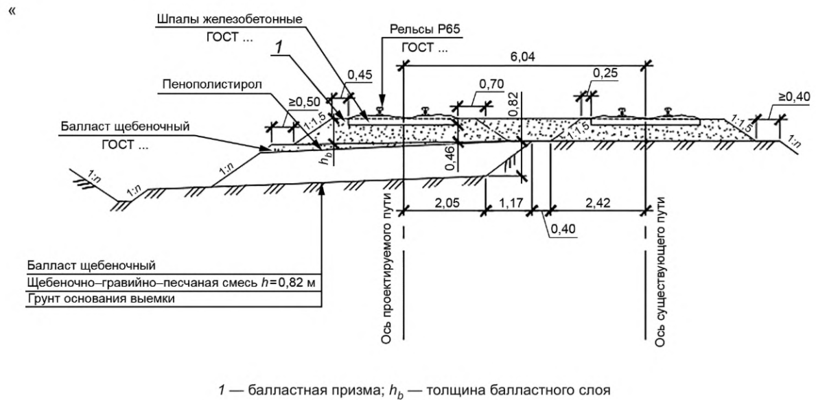
Рисунок П.3 — Конструкция земляного полотна и верхнего строения пути с полузаглубленной балластной призмой».
