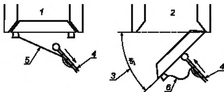
1 — открытие двери; 2 — закрывание двери; 3 — угол открывания; 4 — толкатель; 5 — трос в натянутом состоянии; 6 — трос без натяжения
