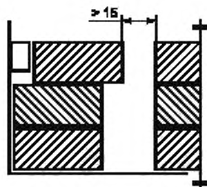
Рисунок 8 — Размещение стопок пакетов, уложенных со смещением
