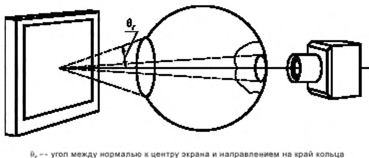
Рисунок 48 — Конфигурация смотрового отверстия/окна
