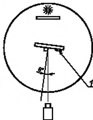
1 — эталон белого
