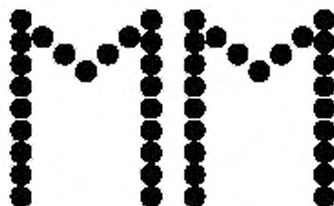
Рисунок 9 — Межзнаковый интервал
