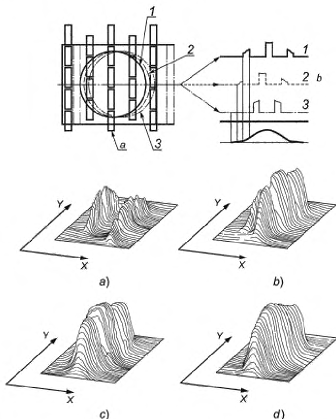
1 — измерение 1; 2 — измерение 2, 3 — измерение 3, на рисунках a)–d) представлена реконструкция распределения яркости за четыре шага; a — отверстие маски; b — средняя линия видеосигнала при измерениях 1-2-3 и комбинации
