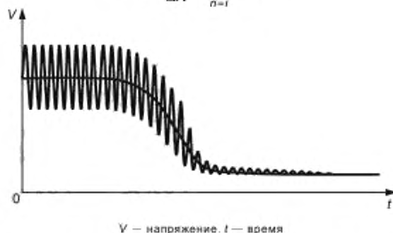
Рисунок 53 — Кривая переходной характеристики (SRF) с периодической пульсацией
